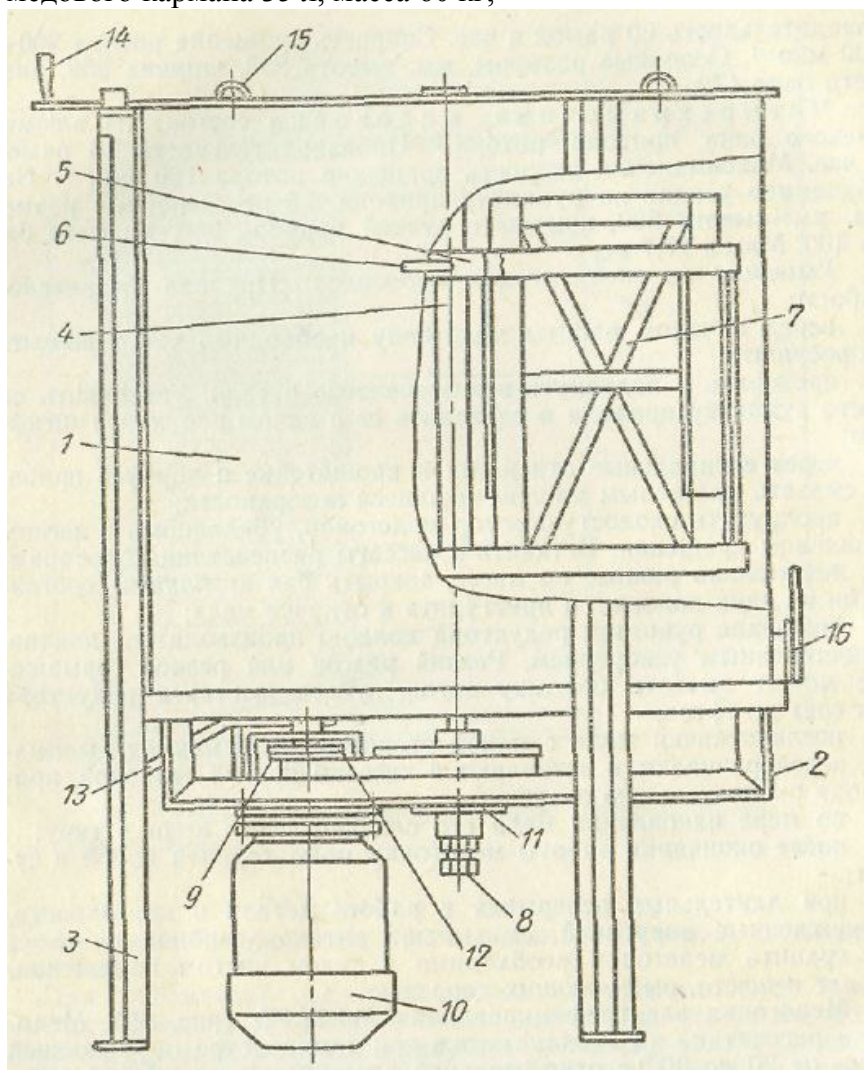
Рис. 32. Схема устройства медогонки электрифицированной М4.32.РЭ
