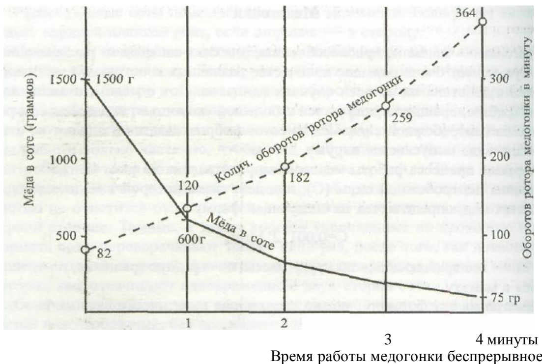
Рис.1. Диаграмма процесса работы радиальной медогонки
