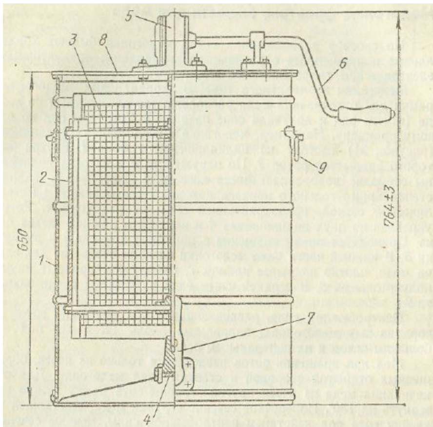
Рис. 1. Схема устройства медогонки трехрамочной хордиальной МЗРС
